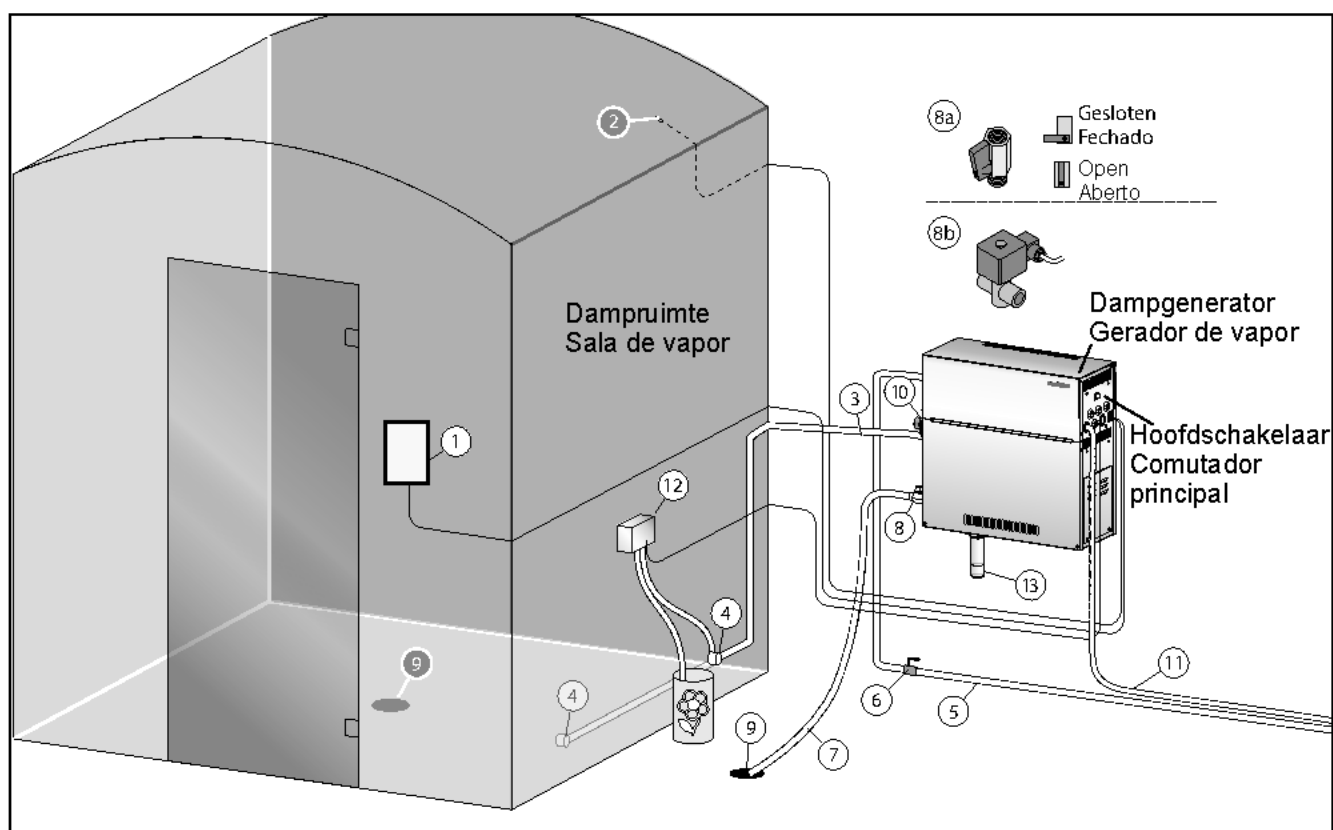
Fig. 1 Systeemonderdelen dampgenerator
