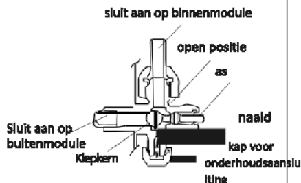
Schema met 3-wegklep
