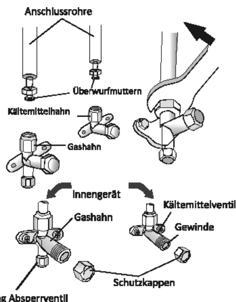
Abdeckung Absperrventil
