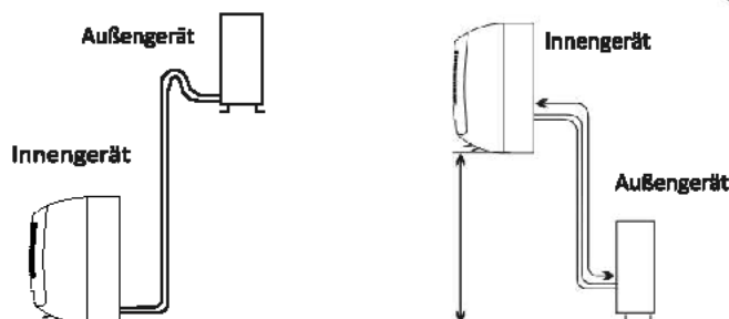
Schaubild zur Installation
