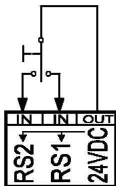
Kuva 6 Etäkäynnistys
