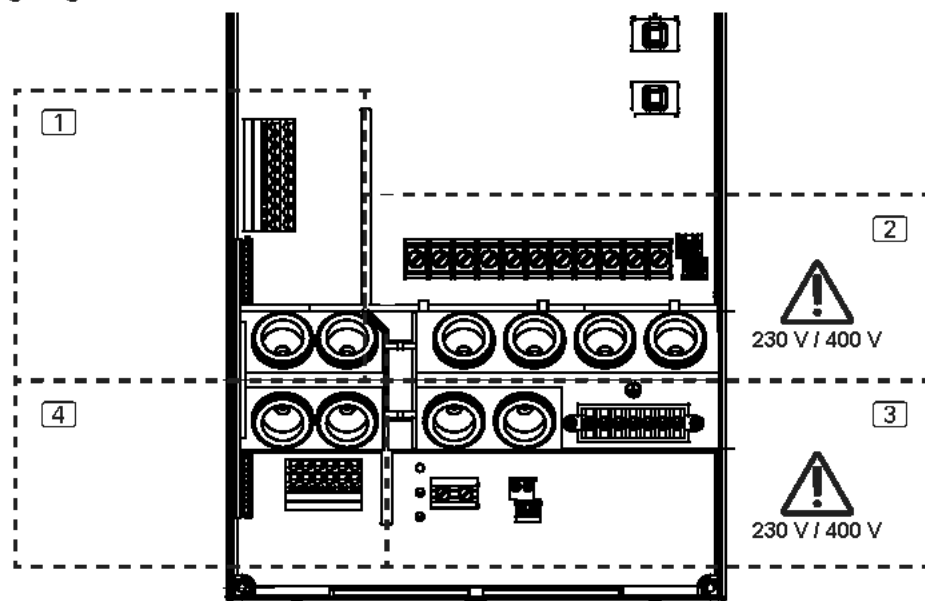
Abb.4 Anschlussbereiche
