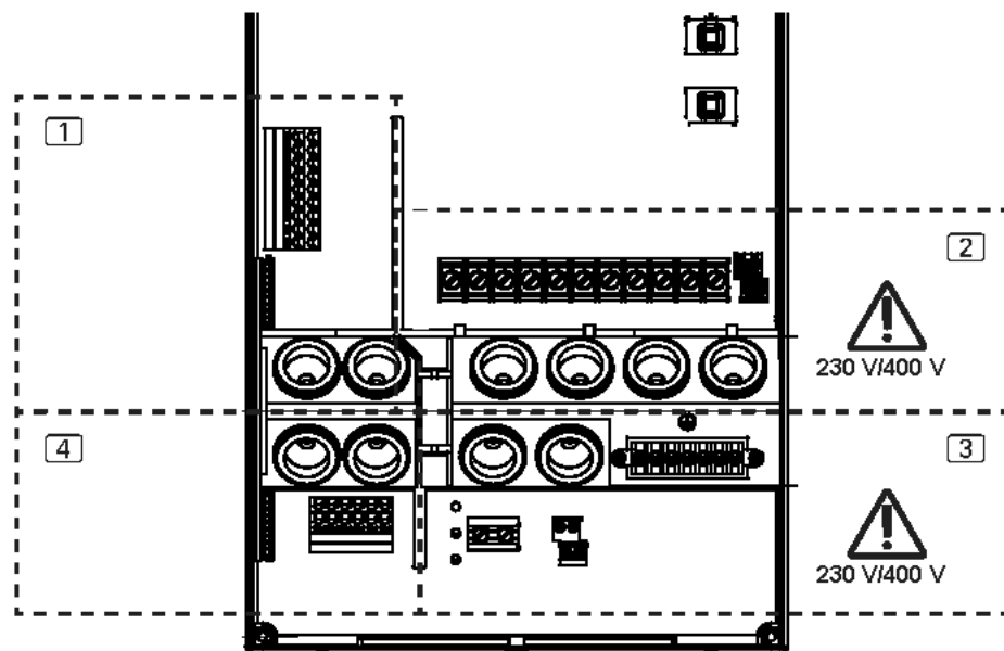
Bild 4 Anslutningsområden
