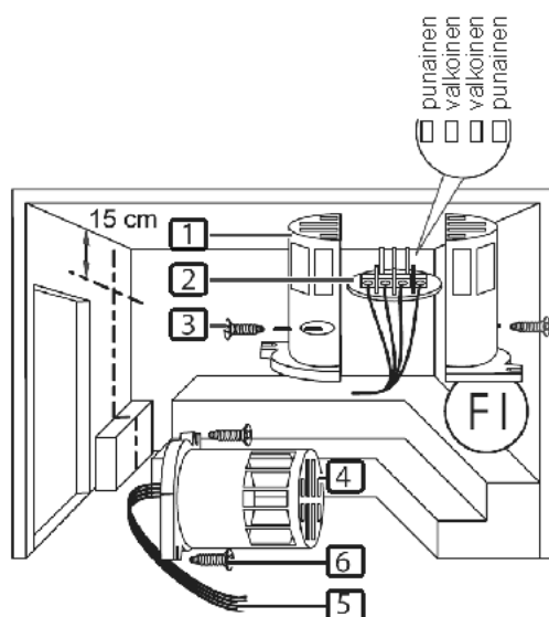
Kuva 5 Kiuasanturin asentaminen
