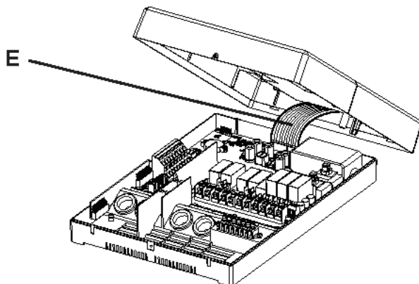
Abb.3 Flachbandkabel ausstecken
