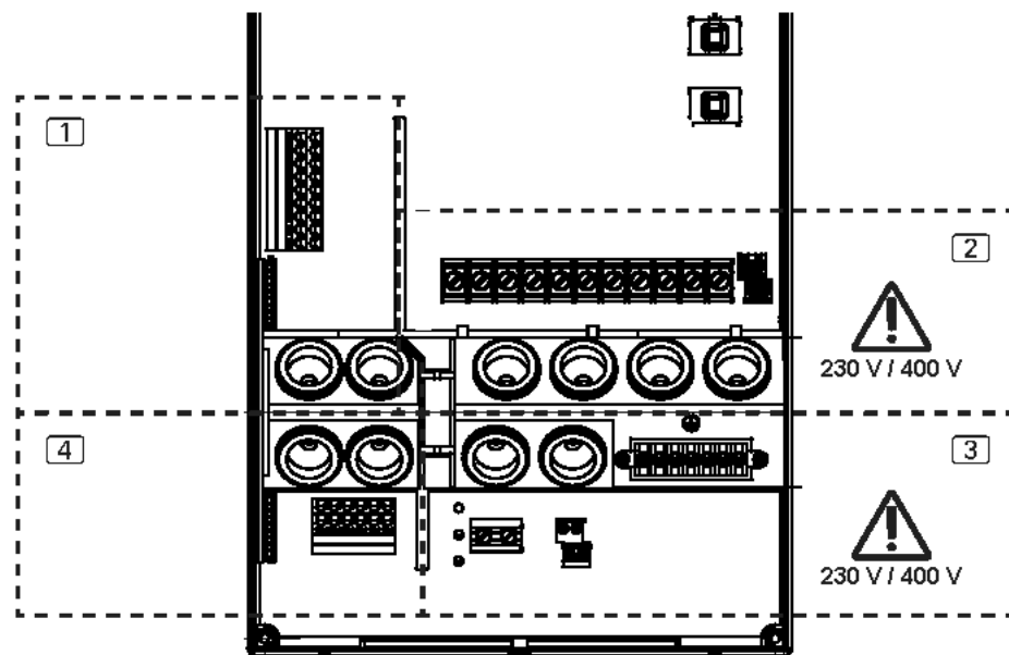
Kuva 4 Liitäntäalueet
