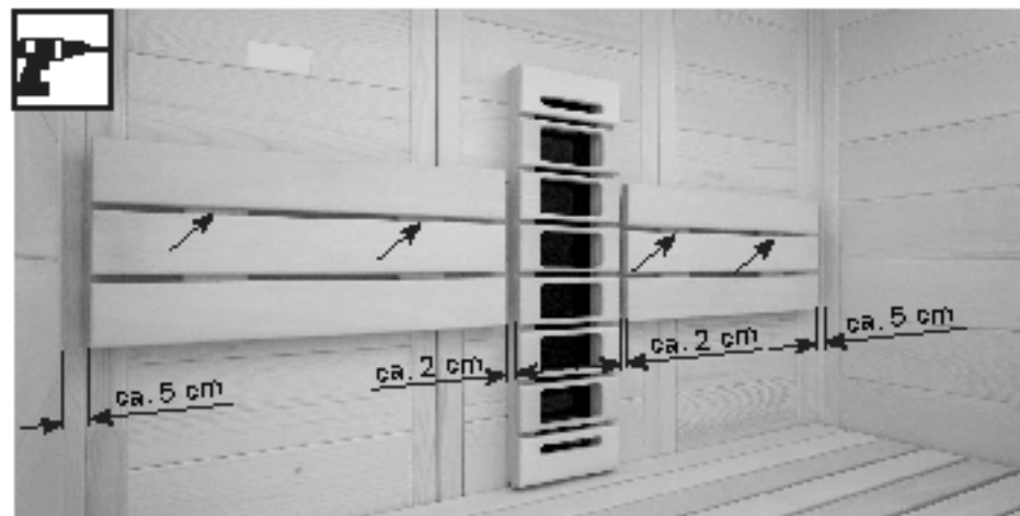
Punta per trapano da 3 mm, 4 viti 4 x 70 mm
