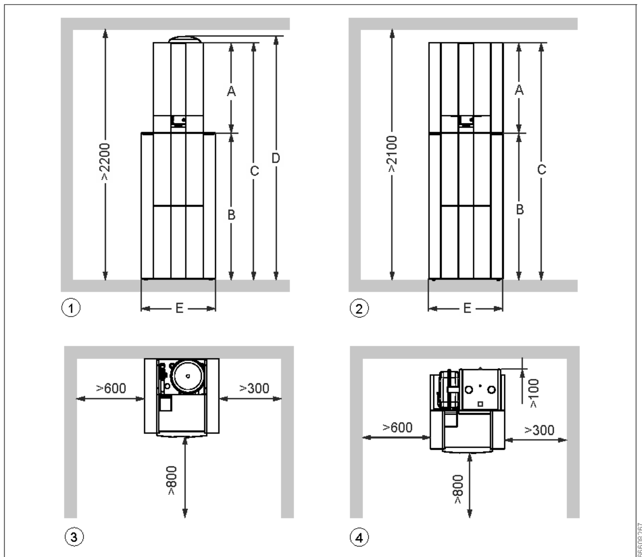
1 Vorderansicht CHC-Monoblock / 200
