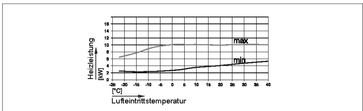
Abb. 13: Heizleistung CHA-10 bei einem Vorlauf von 45 °C
