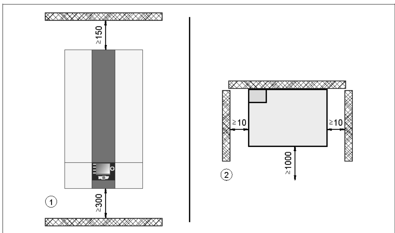
1 Frontansicht IDU
