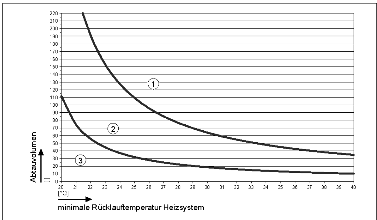
Abb. 4: CHA-10
