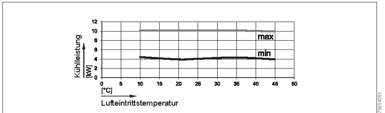
Abb. 18: Kühlleistung CHA-10 bei einem Vorlauf von 18 °C
