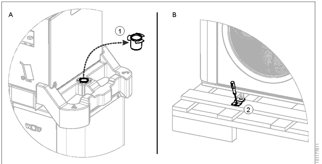
1 Kondensatstutzen
