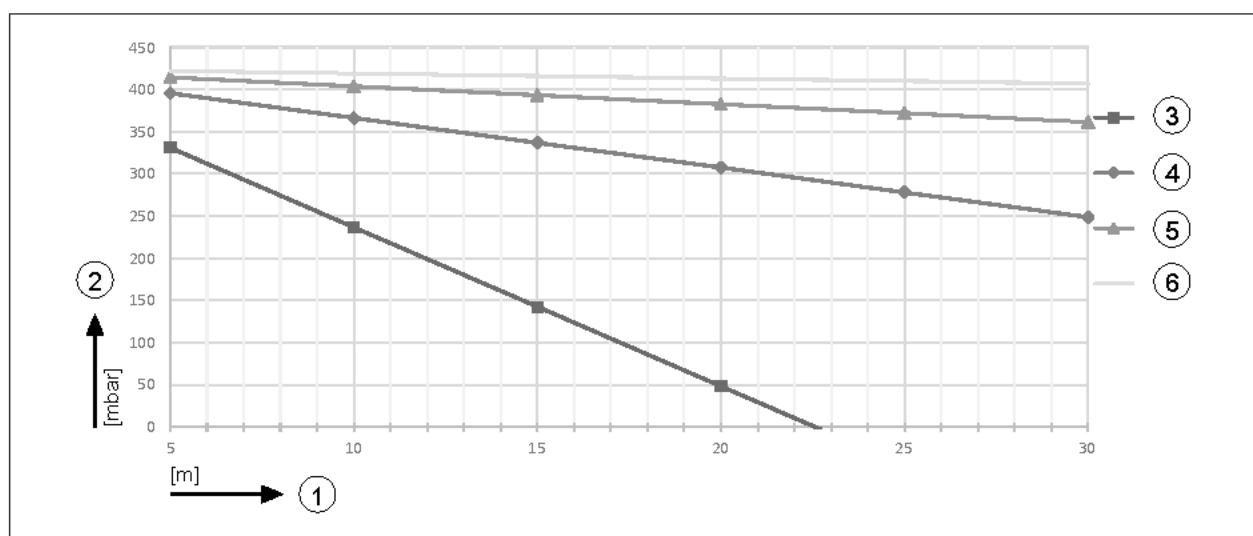
Abb. 1: CHA-07 Verfügbare Förderhöhen
