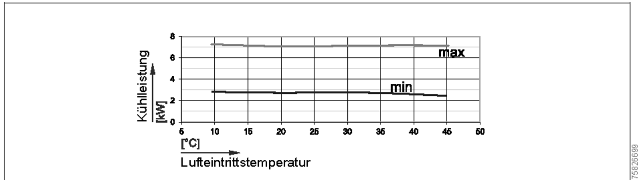
Abb. 16: Kühlleistung CHA-07 bei einem Vorlauf von 18 °C
