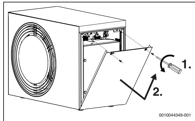
Bild 30 Seitliche Abdeckung
