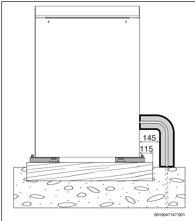
Bild 21 Montageset, Seitenansicht
