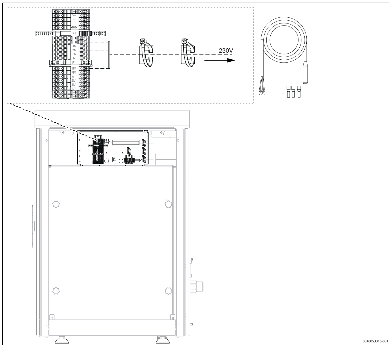
Bild 38 Heizkabelanschluss (Zubehör)
