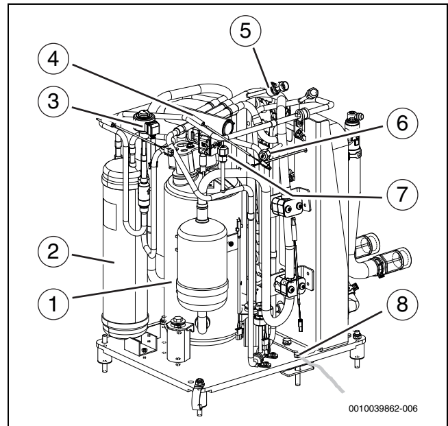
Bild 2 Produktübersicht – Vorderansicht
