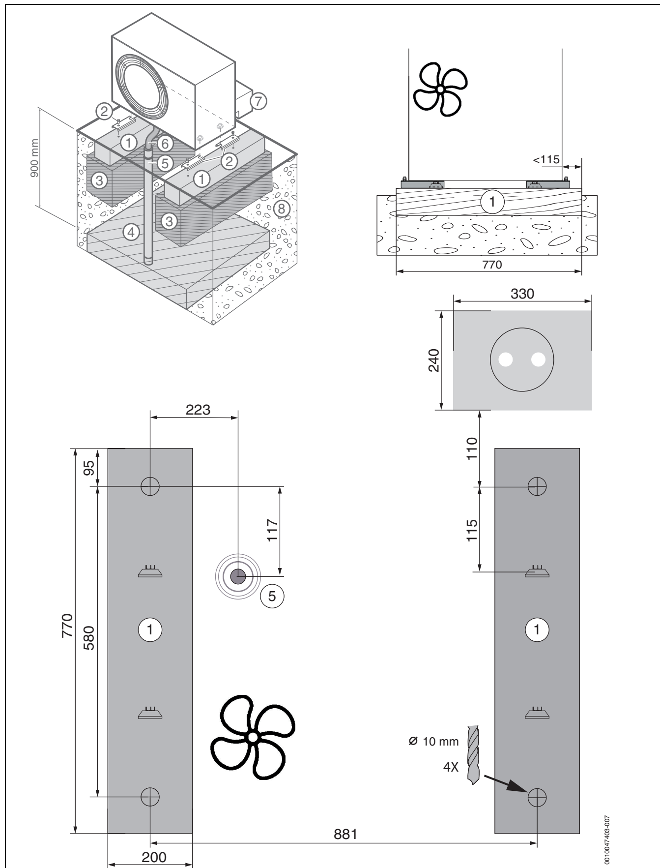
Bild 27 Fundamentplan, Alternative 1
