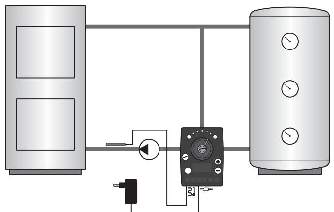
LK 100 in einem Festbrennstoffsystem
