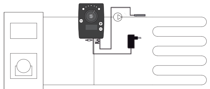
LK 100 in einer Fußbodenheizung
